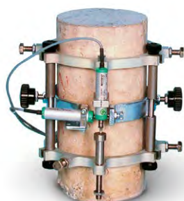
C133N КОМПРЕССОМЕТР/ЭКСТЕНЗОМЕТР
