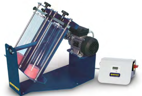
A080 КИТ УДАРНЫЙ ИСПЫТАТЕЛЬНЫЙ АППАРАТ
